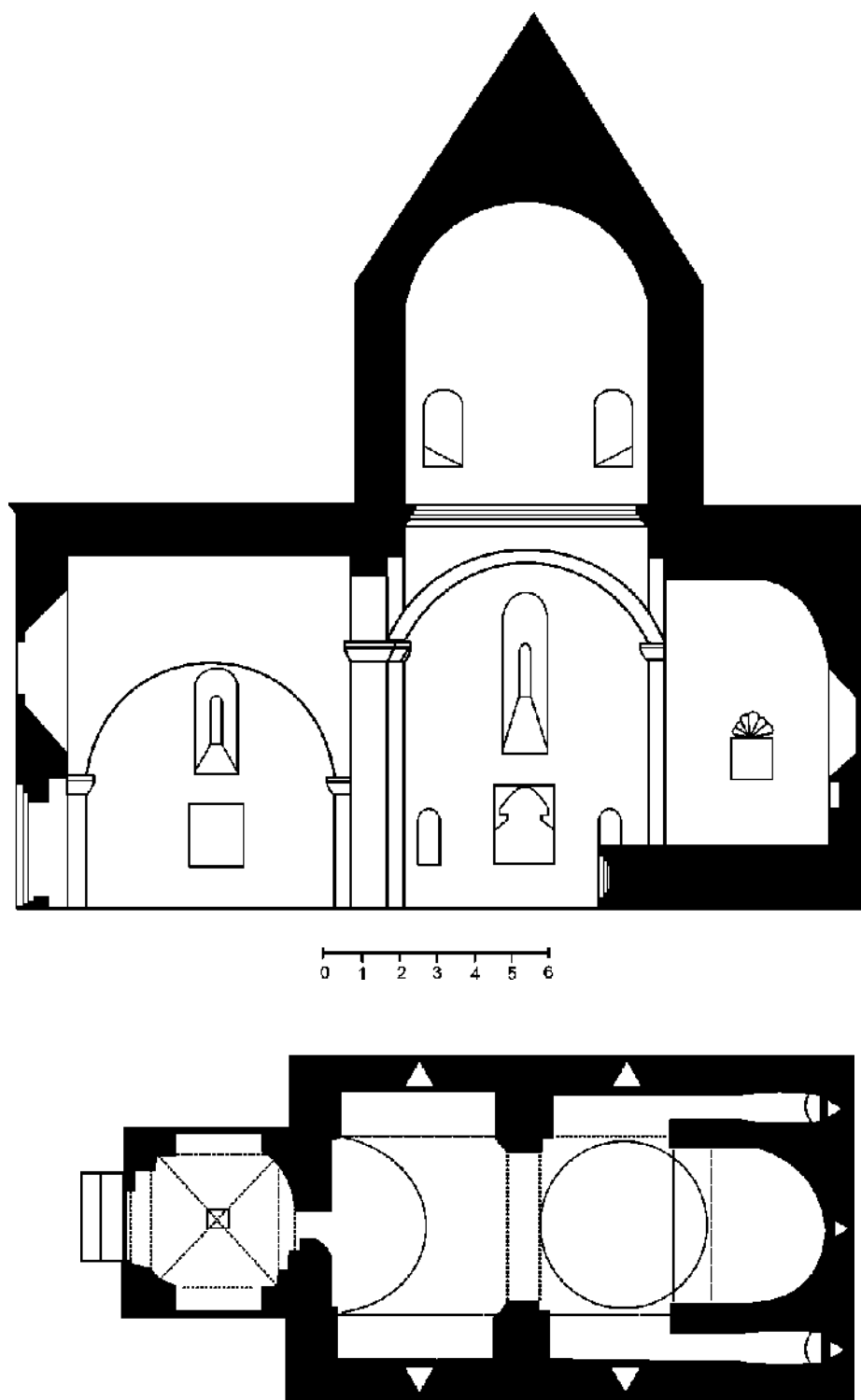
Գծանկ. 2ա, 2բ Ս. Աստվածածին եկեղեցու կտրվածքն ու հատակագիծը (արտատպված՝ «Նյութեր Կովկասի հնագիտության» (MAK) ժողովածուից, հատակագիծը՝ Մ. Հասրաթյանի)
