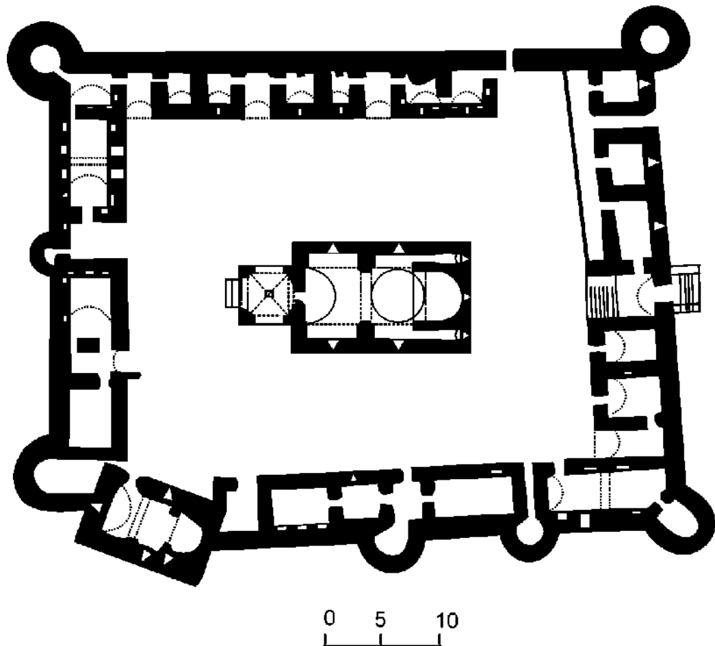
Գծանկ. 3 Խոր Վիրապ վանական համալիրի գլխավոր հատակագիծը (ըստ Մ. Հասրաթյանի)
