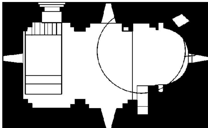
Գծանկ. 1ա, 1բ Ս. Գրիգոր Լուսավորիչ եկեղեցու և Ս. Վիրապի կտրվածքն ու հատակագիծը (արտատպված՝ «Նյութեր Կովկասի Հնագիտության» (MAK) ժողովածուից)
